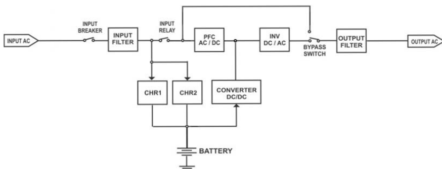
شکل ۲۵: ساختار داخلی یوپی‌اس‌های SDC2000-PF1 و SDC1500X-RT
