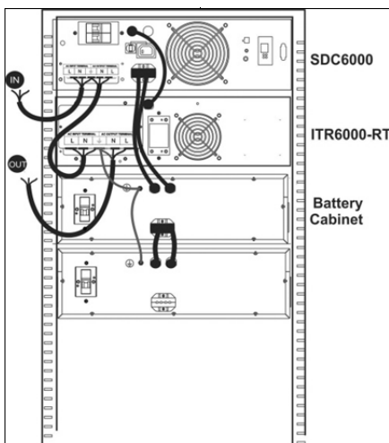
شکل ۱۴- ب: یوپی اس SDC6000، ترانسفورمر ایزوله و دو کابینت باتری
