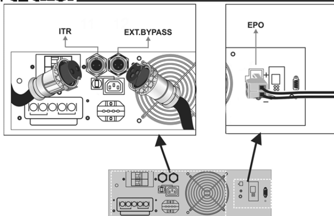
شکل ۲۴: شکل پنل پشت و اتصالات مربوط به ترانسفورمر ایزوله، تابلوی بای‌پس و EPO
