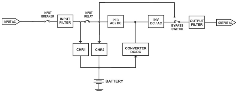
شکل ۲۷: ساختار داخلی یوپی‌اس‌های SDC3000X-RT و SDC2000X-RT
