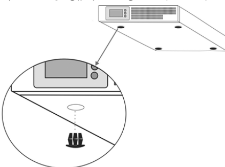
شکل ۱۱: قرار دادن پین‌های پولکی
