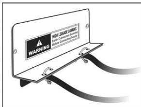
شکل ۲۳: نحوه‌ی محکم کردن کابل‌ها به درپوش L شکل ترمینال ورودی-خروجی
