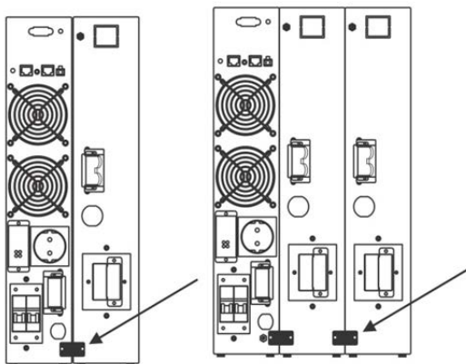
شکل ۱۸: نحوه قرار گرفتن بست‌های نگهدارنده در پشت یوپی‌اس و کابینت باتری
