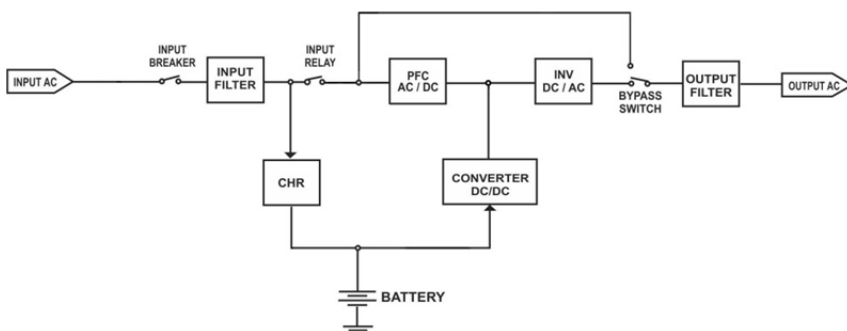
شکل ۲۶: ساختار داخلی یوپی‌اس‌های SDC1500BW
