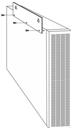
شکل ۲۰: مونتاژ قطعه آویز به SDC1500BW
