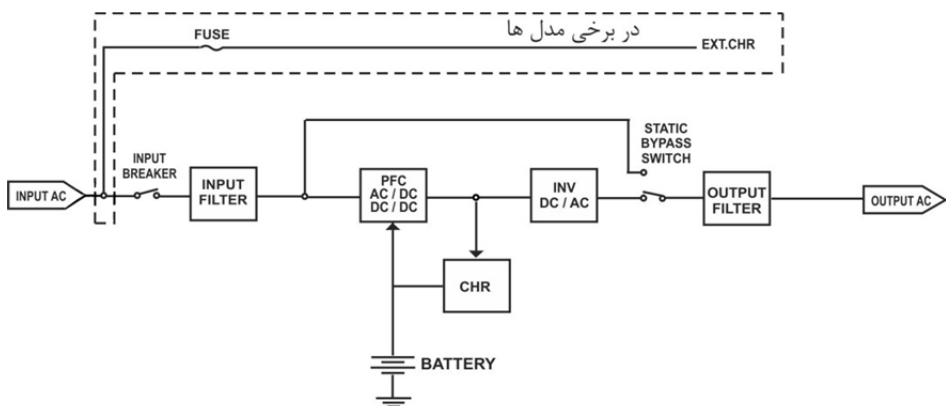
شکل ۲۸: ساختار داخلی یوپی‌اس‌های SDC6000X-RT
