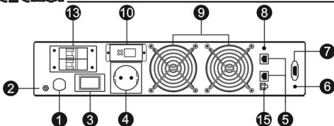
شکل ۳: نمای پنل پشت SDC مدل (RT-2U)
