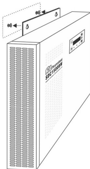
شکل ۲۱: نصب SDC1500BW بر روی دیوار
